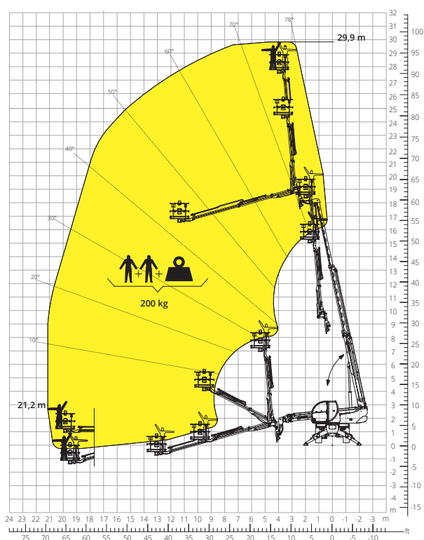
Diagram draagvermogens met TELESCOPISCH WERKPLATFORM 200 kg - 10 m ATT - 01 - 022
