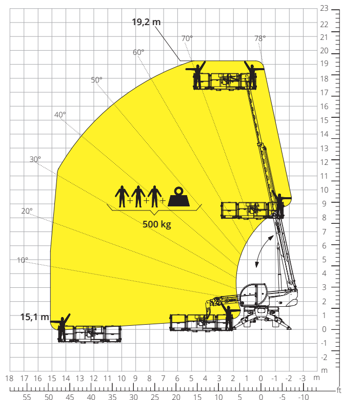
Diagram draagvermogens met ROTEREND UITKLAPBAAR WERKPLATFORM 500 kg ATT-01-007
